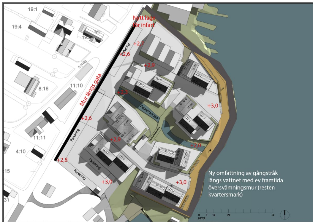
Figur 4: Rekommenderad höjdsättning för avledning av dagvattnet inom planområdet.
